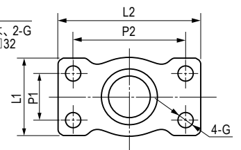
TCA-420R-□50~75
