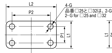
TCA-420R-□25~38
