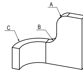
最小曲げ半径説明図 Minimum Bending Radius
