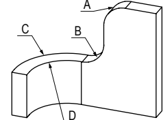
最小曲げ半径説明図 Minimum Bending Radius
