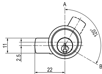
左付の場合 For a left side lock
