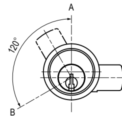
右付の場合 For a right side lock
