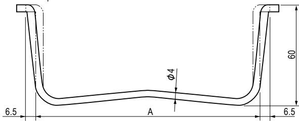
TM-75 スタンドホルダー Stand Holder 2-φ3.1
