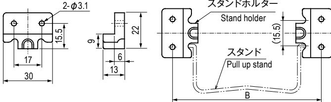
TM-75 スタンドホルダー Stand Holder 2-φ3.1
